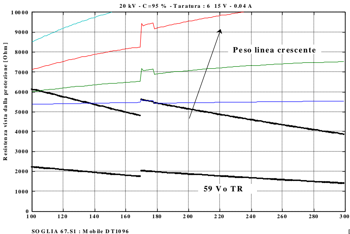
Figura 3: resistenza di guasto a terra selezionabili dalle protezioni di linea MT in regime di esercizio a neutro isolato
